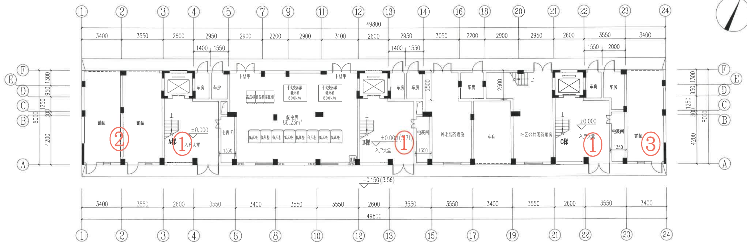
第三幢住宅楼首层平面图
