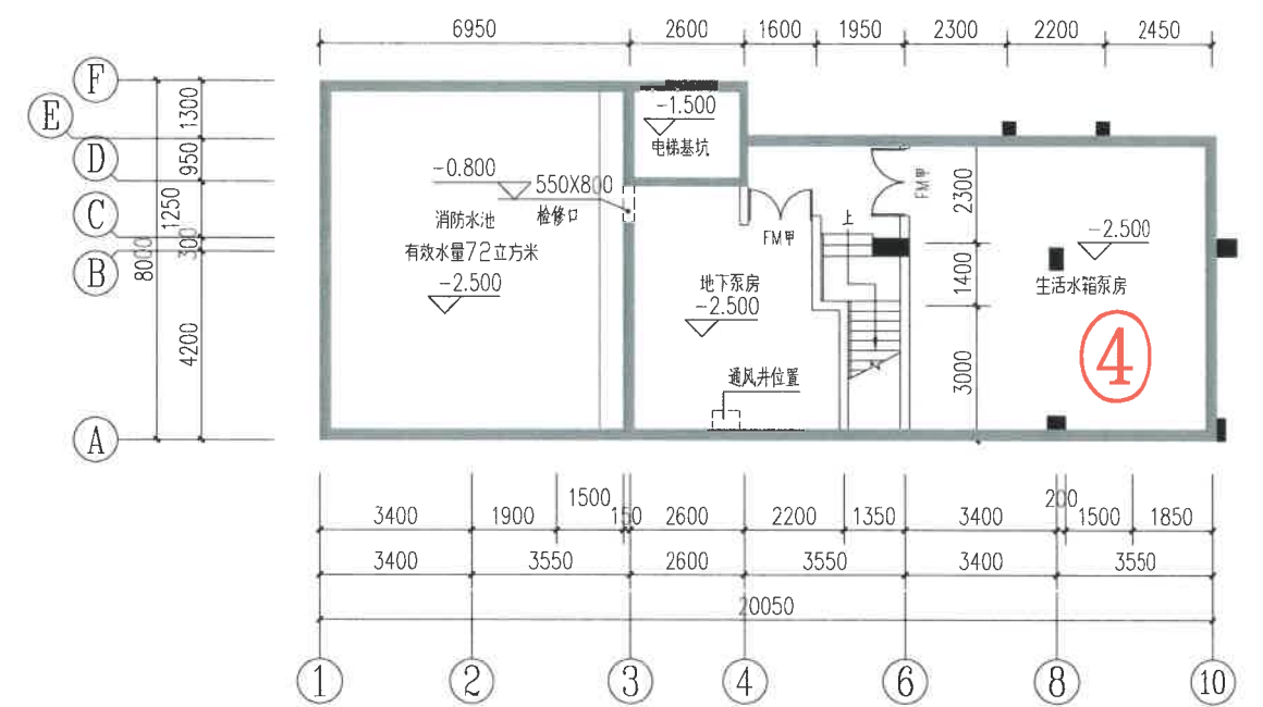
第一幢住宅楼消防水池、生活水箱泵房平面图
