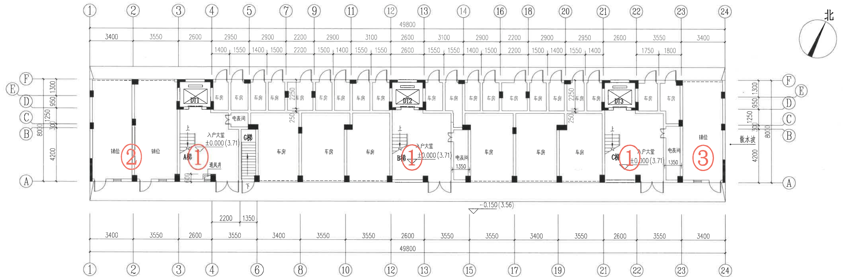
第一幢住宅楼消防水池、生活水箱泵房平面图
