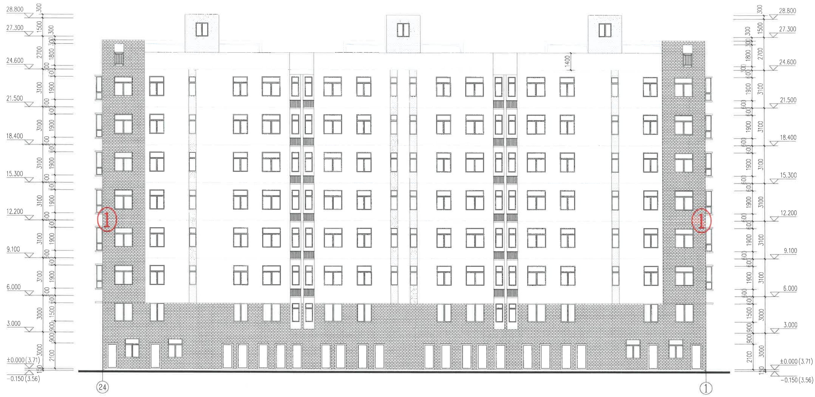
第一幢住宅楼 ②4-①轴立面图
