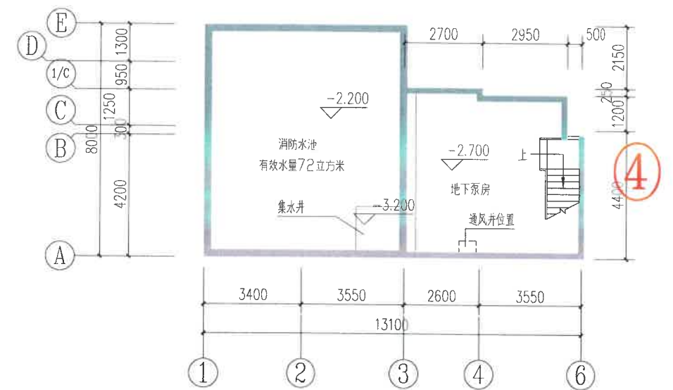
第一幢住宅楼消防水池平面图
