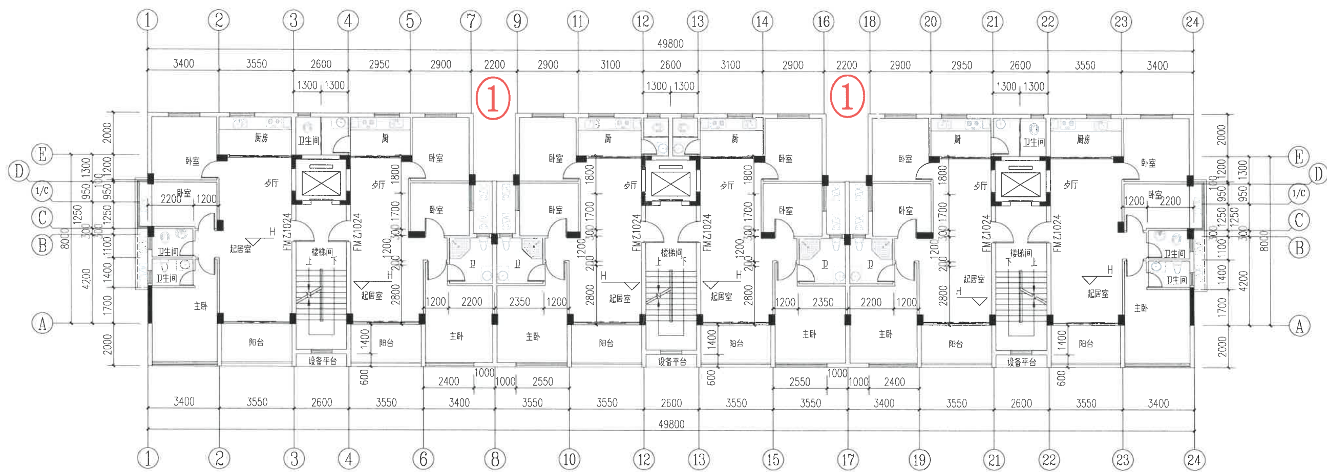
第一幢住宅楼三层平面图
