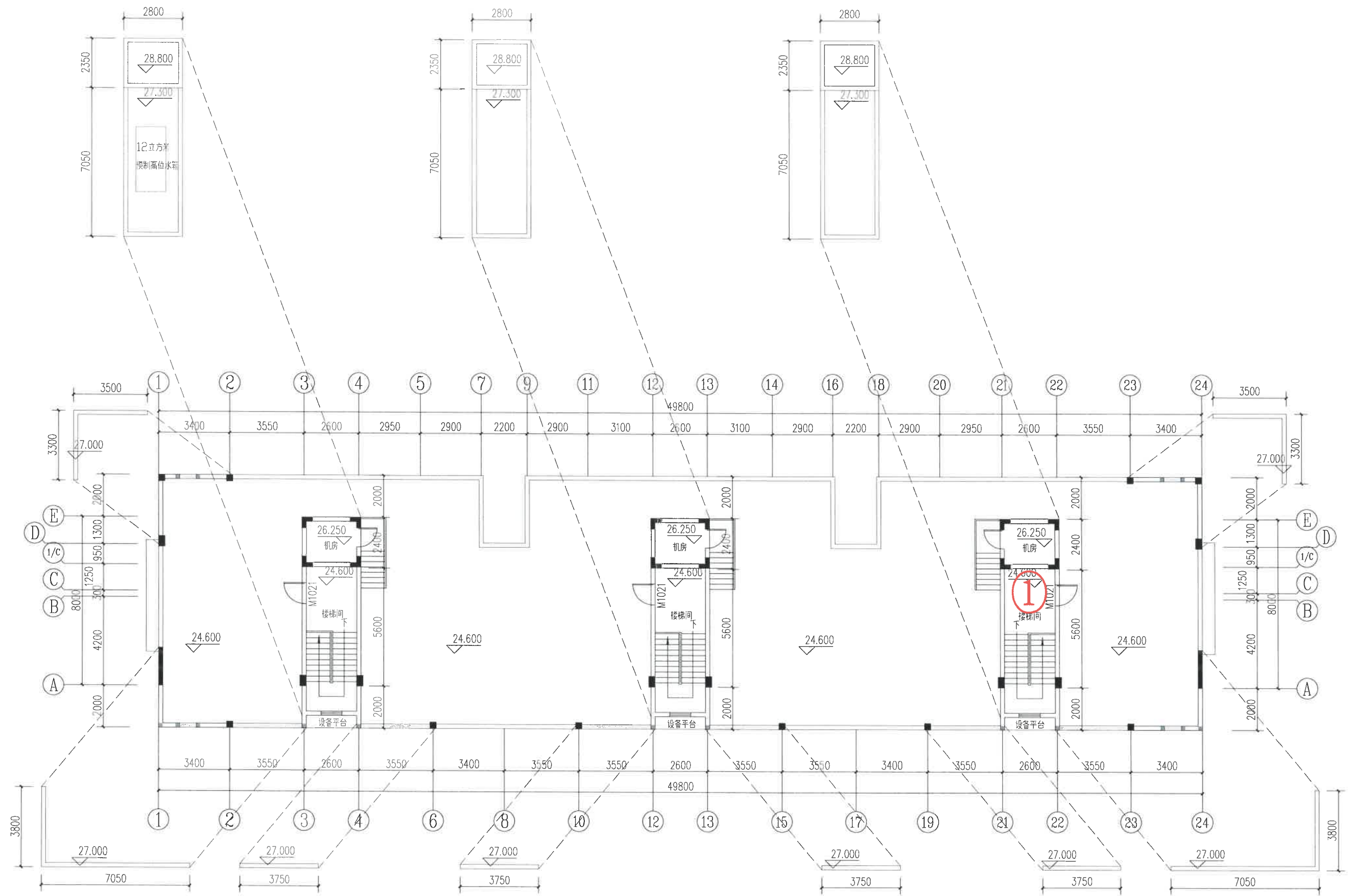
第一幢住宅楼天面平面图
