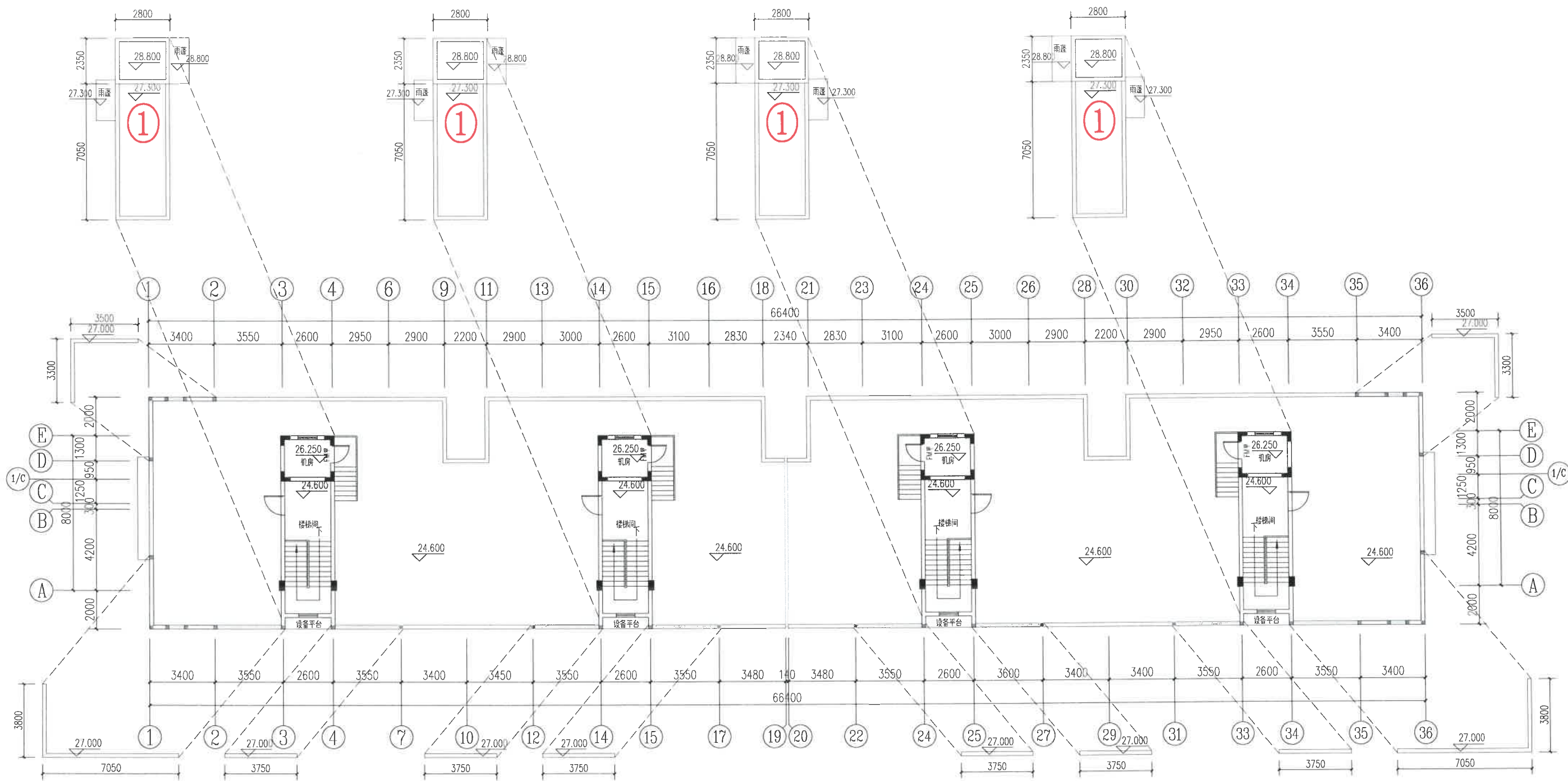
第二幢住宅楼天面平面图
