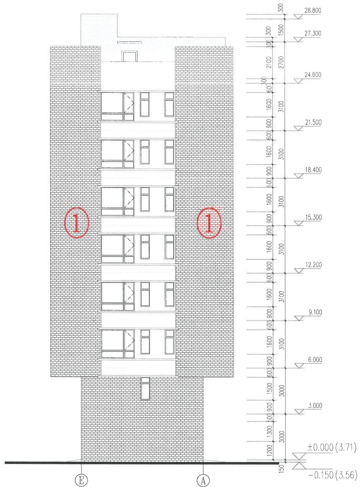
第二幢住宅楼 E-A 轴立面图
