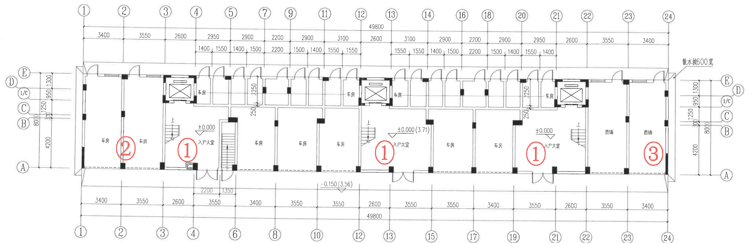
第一幢住宅楼首层平面图
