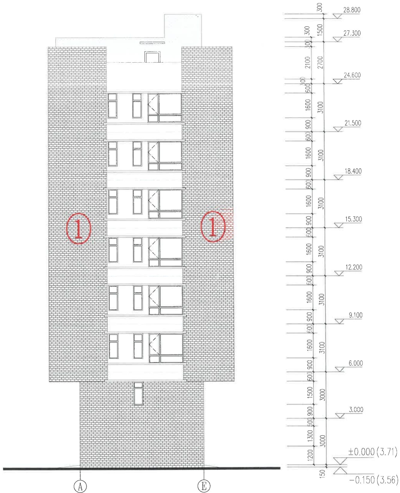
第二幢住宅楼 A-E 轴立面图
