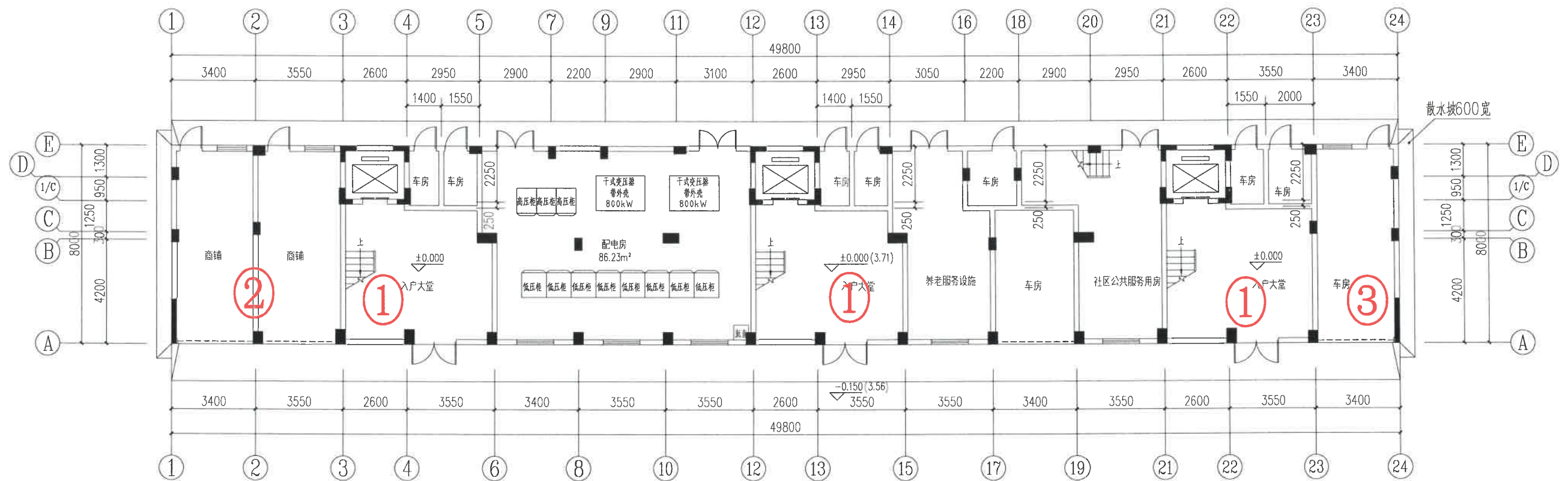
第三幢住宅楼首层平面图
