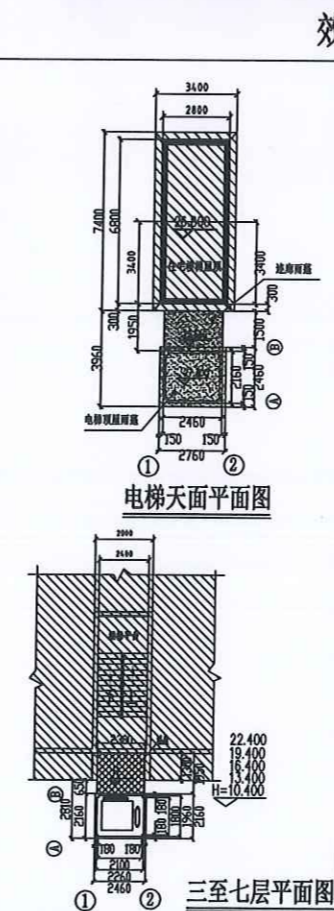
平面图2
