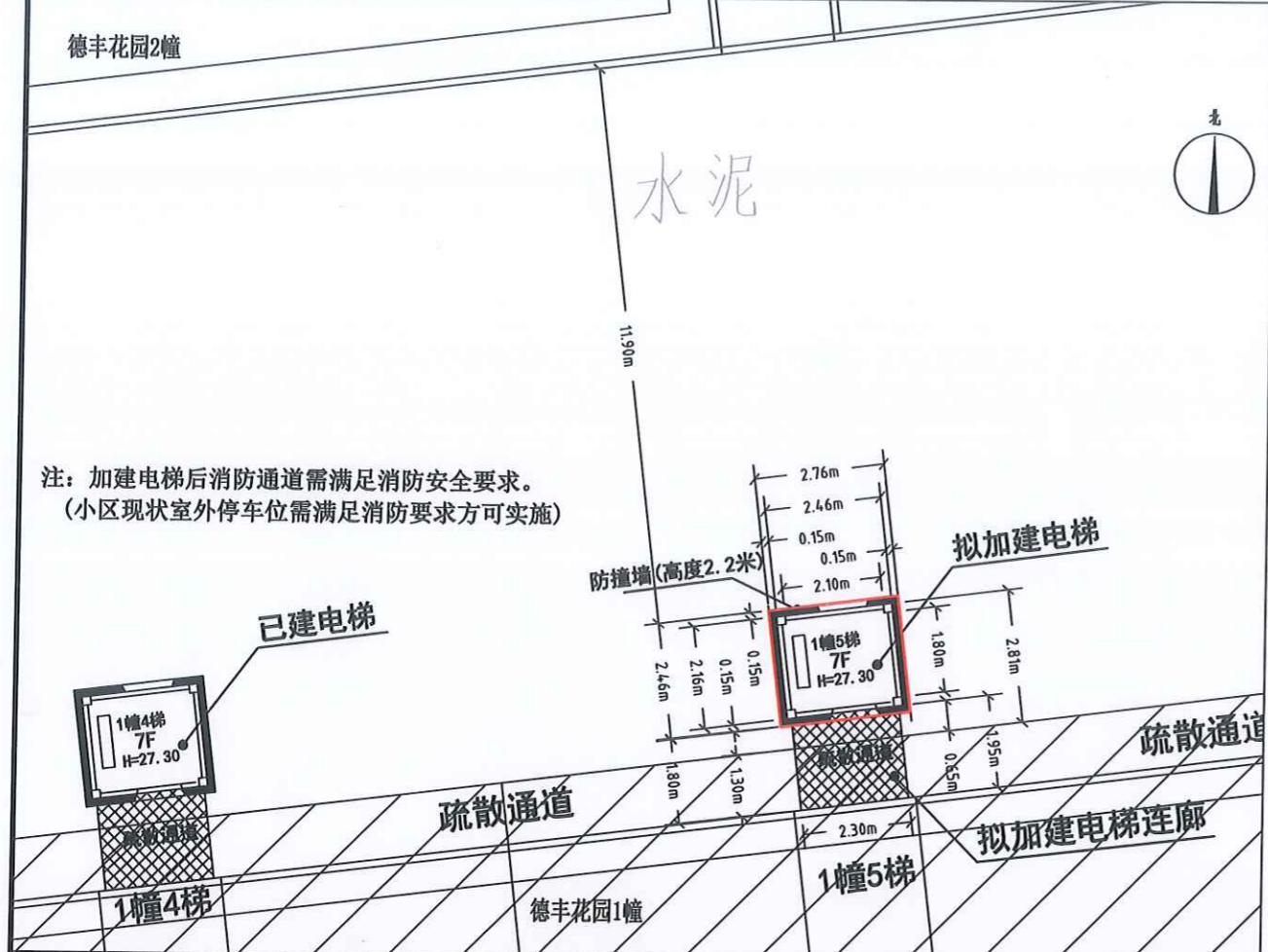
总平面图
