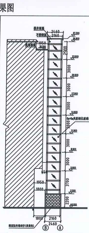
B-A轴立面图
