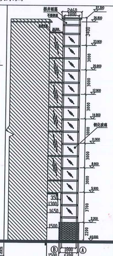
B-A轴立面图
