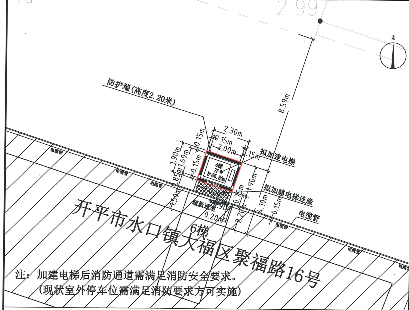
总平面图
