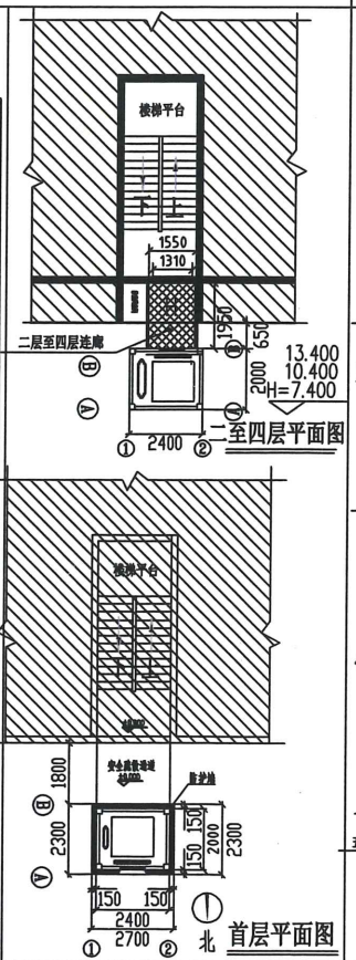
平面图1
