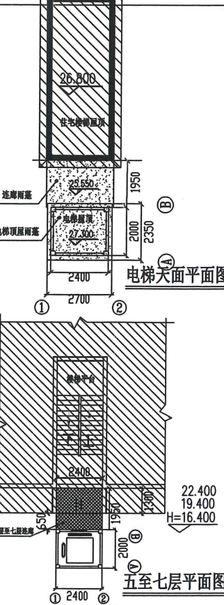
平面图2
