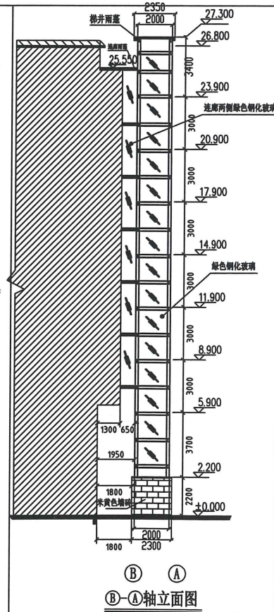
B-A轴立面图
