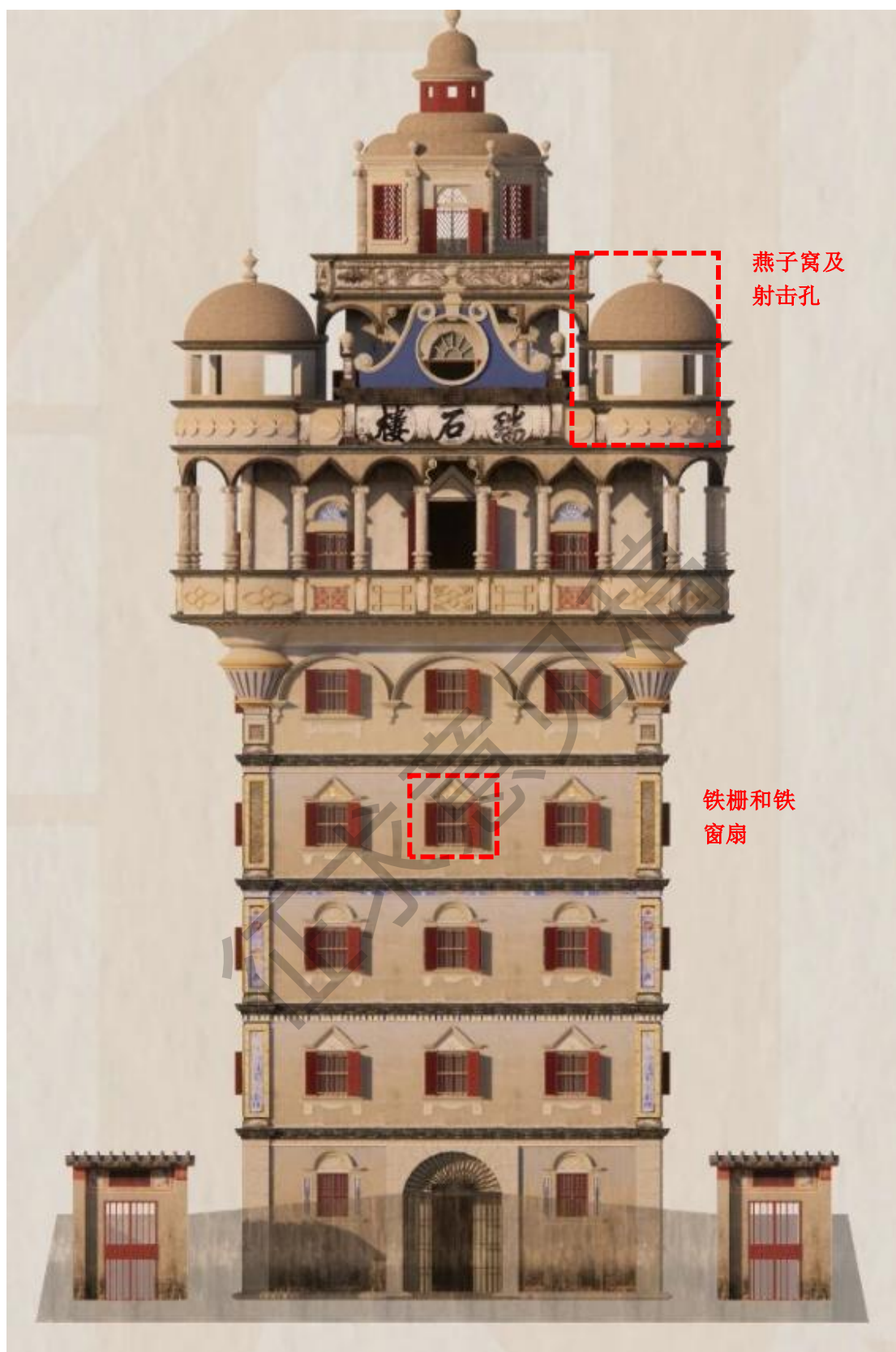
瑞石楼正立面防御构造 14
