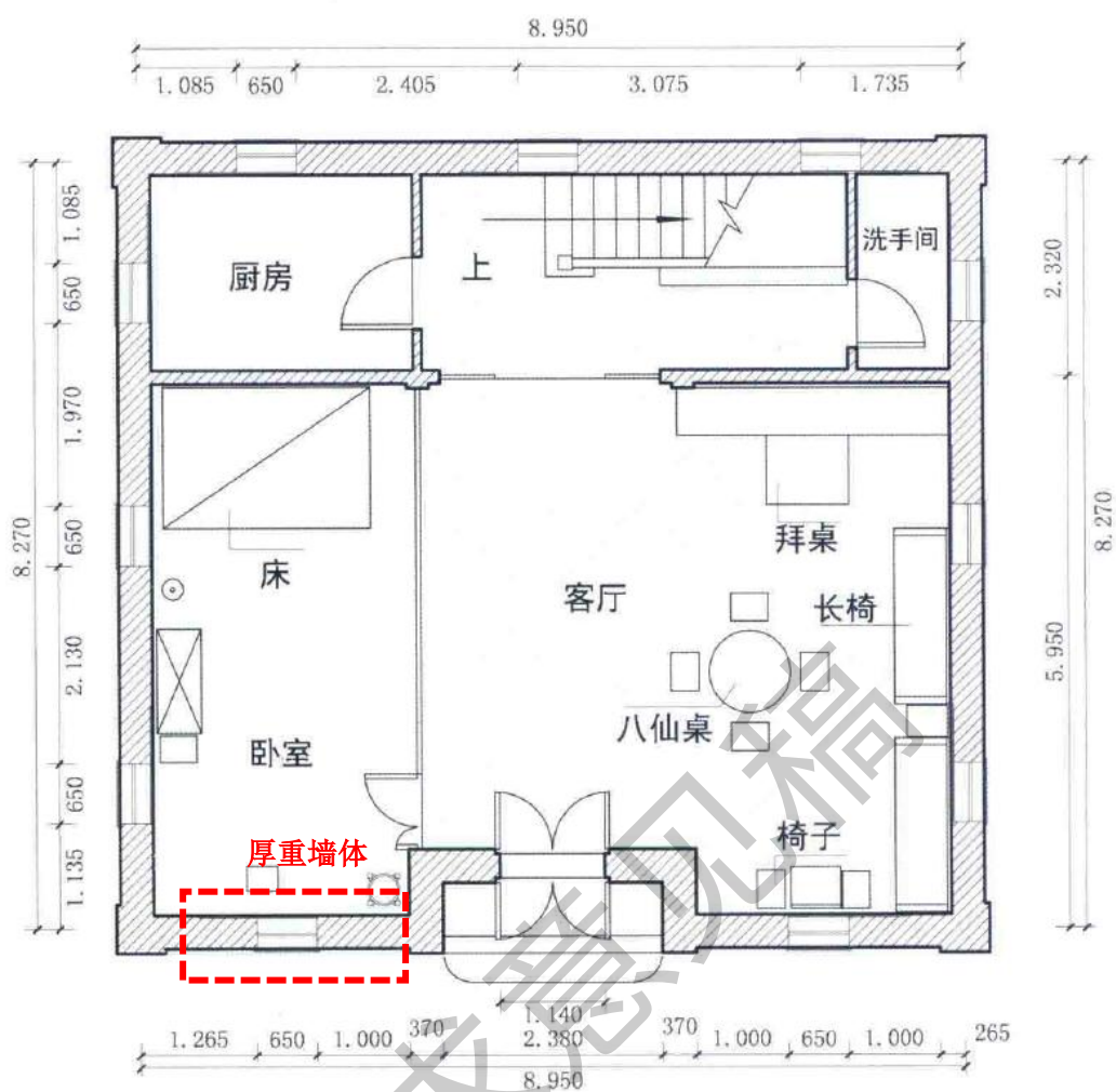
瑞石楼平面防御构造 16
